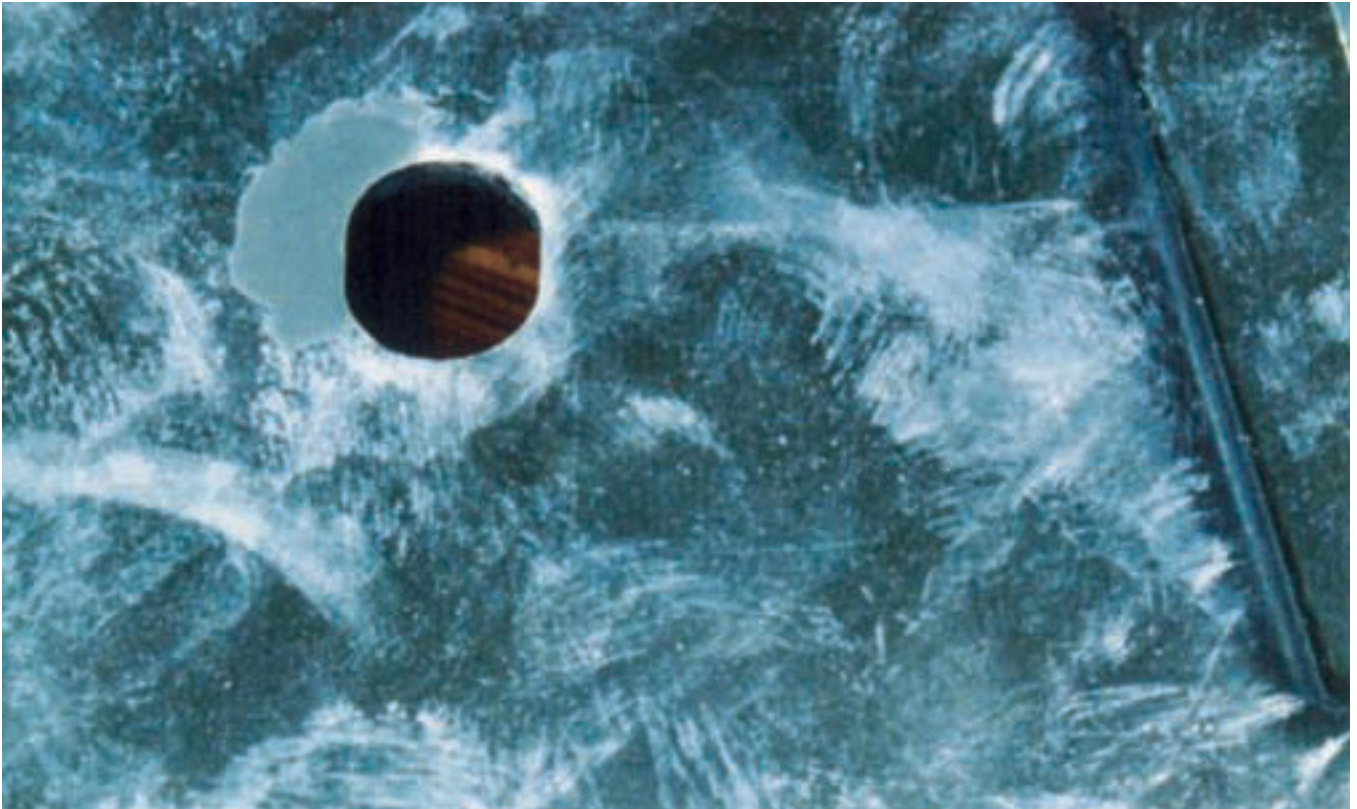
Eksempel på reparation af zinkafskalning omkring et udstanset hul i varmforzinket plade. Reparationen er udført med zinkstøvmaaling.
